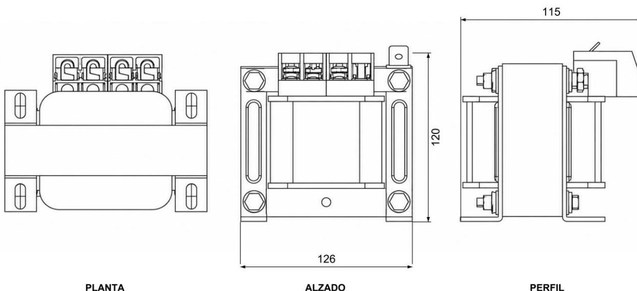
PLANTA
